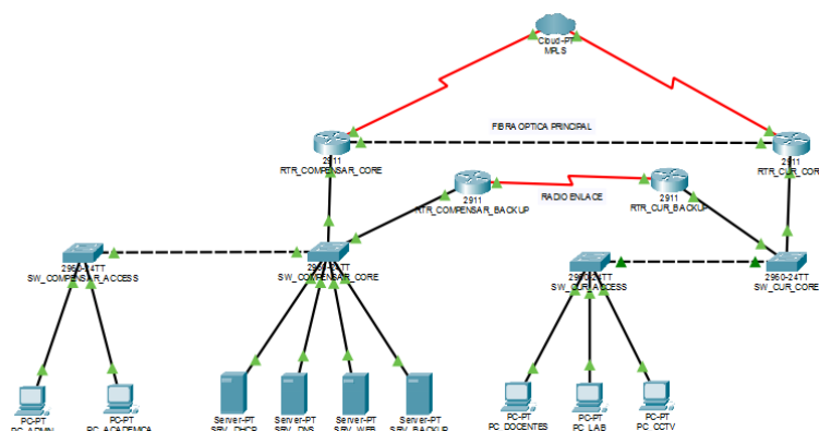
Figura N21 Montaje de conexión entre la infraestructura de la fundación universitaria compensar y la c.u.r compensa
