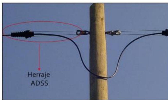
Figura N2 Herraje de retención para cables ADSS
