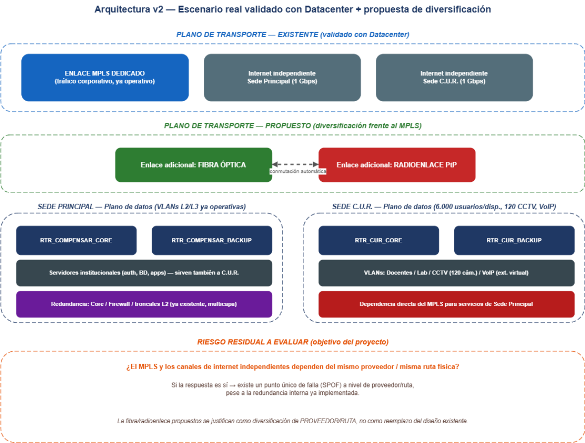
Figura N7 Escenario real validado (MPLS + redundancia existente) y propuesta de diversificación.
