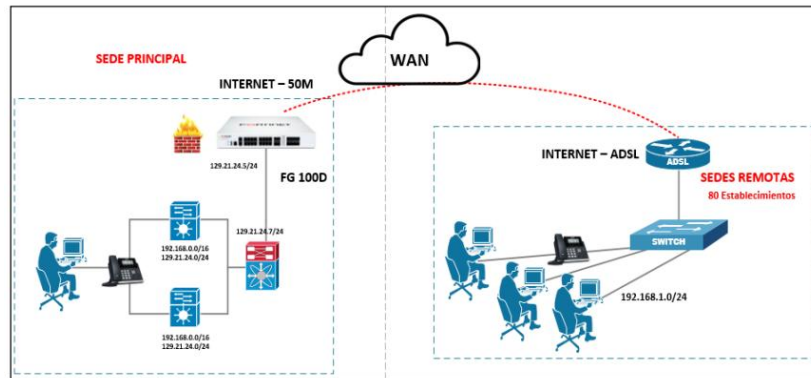
Figura N5 Diagrama de red Lima Este
