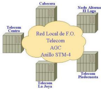
Figura N3 Red local de fibra(Anillo de grandes clientes)
