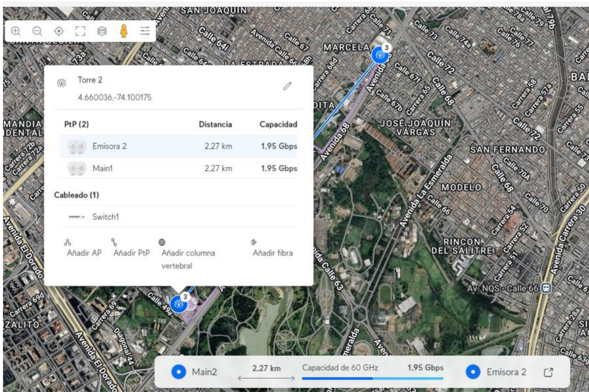
Figura N15 Disponibilidad y alcance de comunicación
