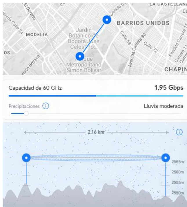
Figura N8 Radioenlace de las dos torres.
